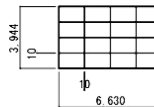
設置概要図 1/200
