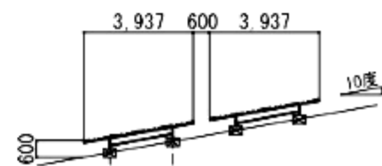
設置概要図 1/200
